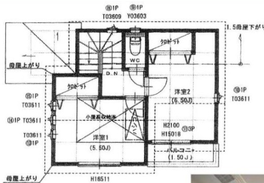
※図面と現況が異なる場合は現況優先といたします。 2階平面図
